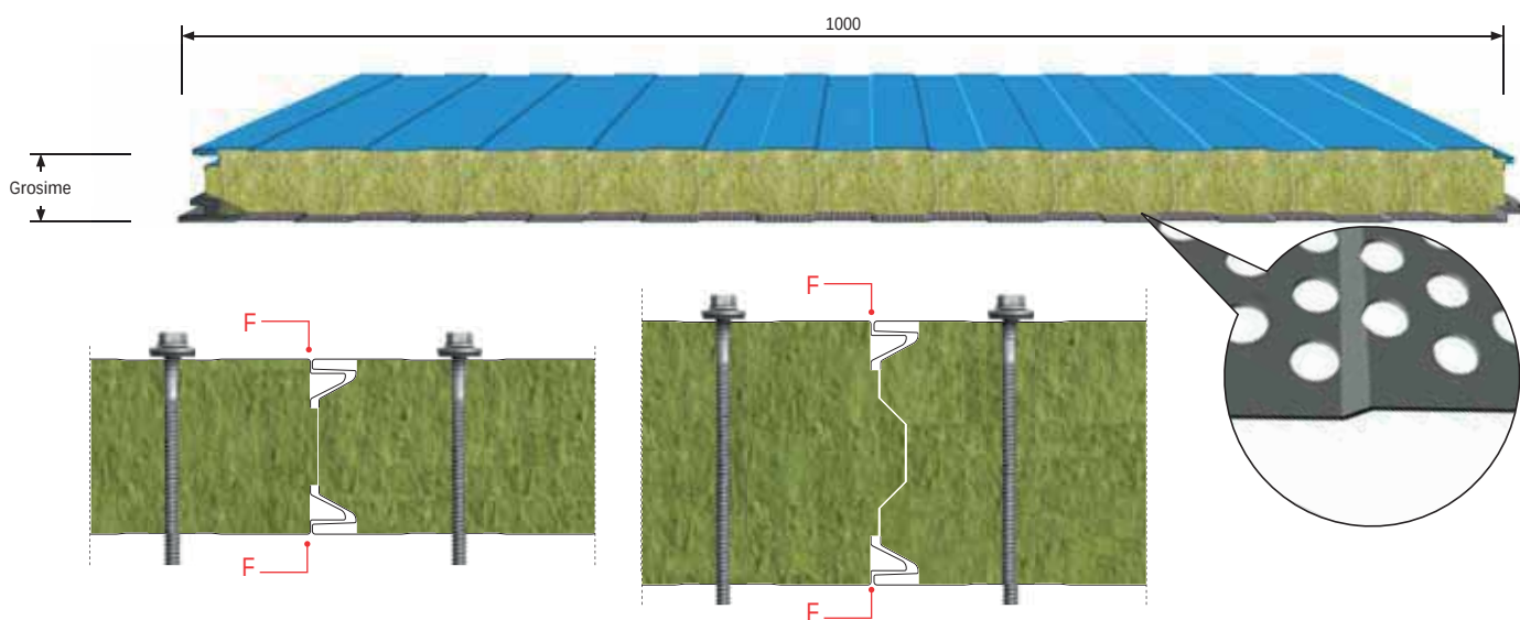
Detaliu îmbinare
