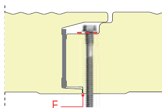
Detaliul - Isopan Iberica (Spania)
