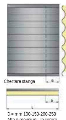
Detaliul sistemului de chertare
