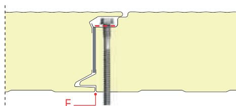
Detaliul - Isopan Spa (Italia)
