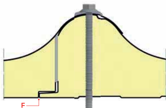
Detaliul sistemului de cuplare și încastrare
