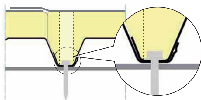
Detaliu sistem de fixare
