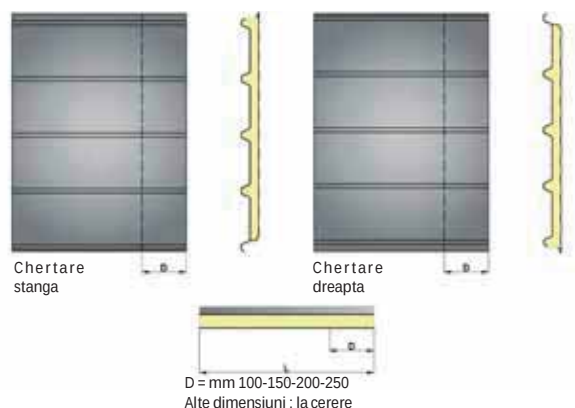
Detalii sistemului de chertare
