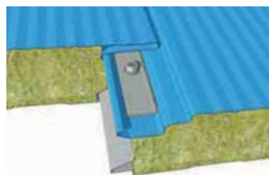
Utilizare in pozitie orizontala
