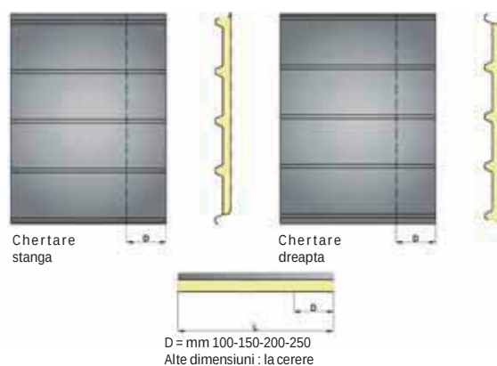
Detalii sistemului de chertare
