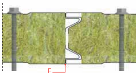
Detaliu îmbinare
